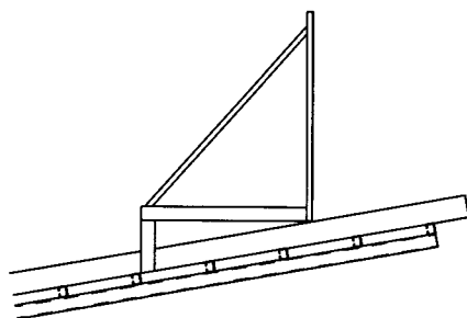
④ 庇の上の看板 J R 博多駅筑紫口 P 案内 (当社による構造計算)
