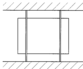
④ 上下固定式看板 J R 小倉駅新幹線高架内 (当社による構造計算)
